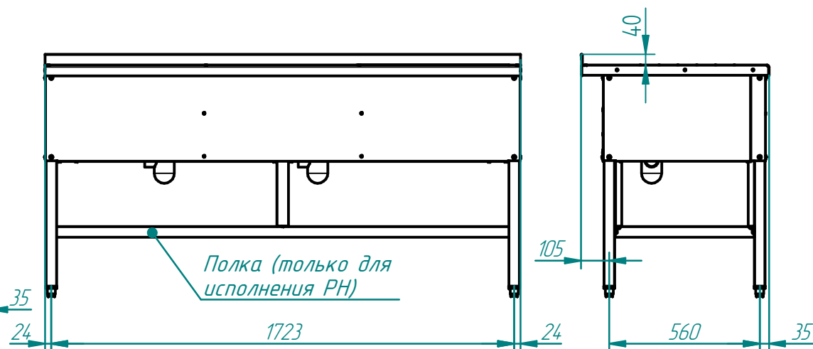
СМО-7-7 РН и СМО-7-7 РЧ
