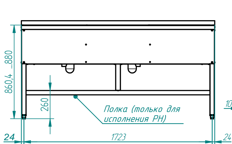
СМО-6-7 РН и СМО-6-7 РЧ
