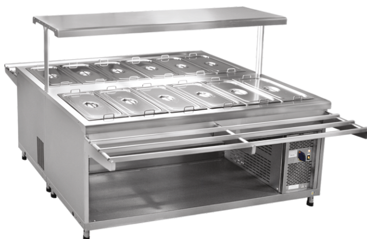
ПВВ(Н)-140СМ-02
